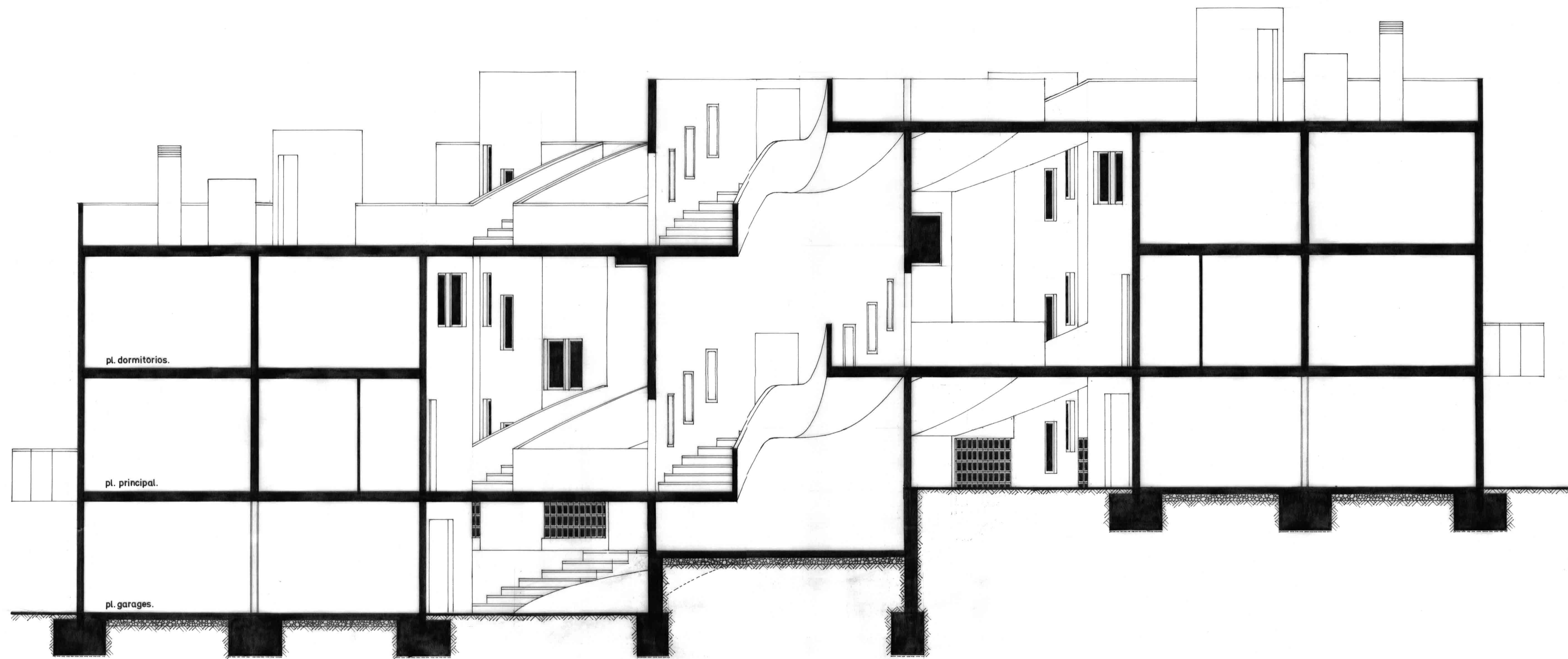
sección a-a'. e-1:50.
