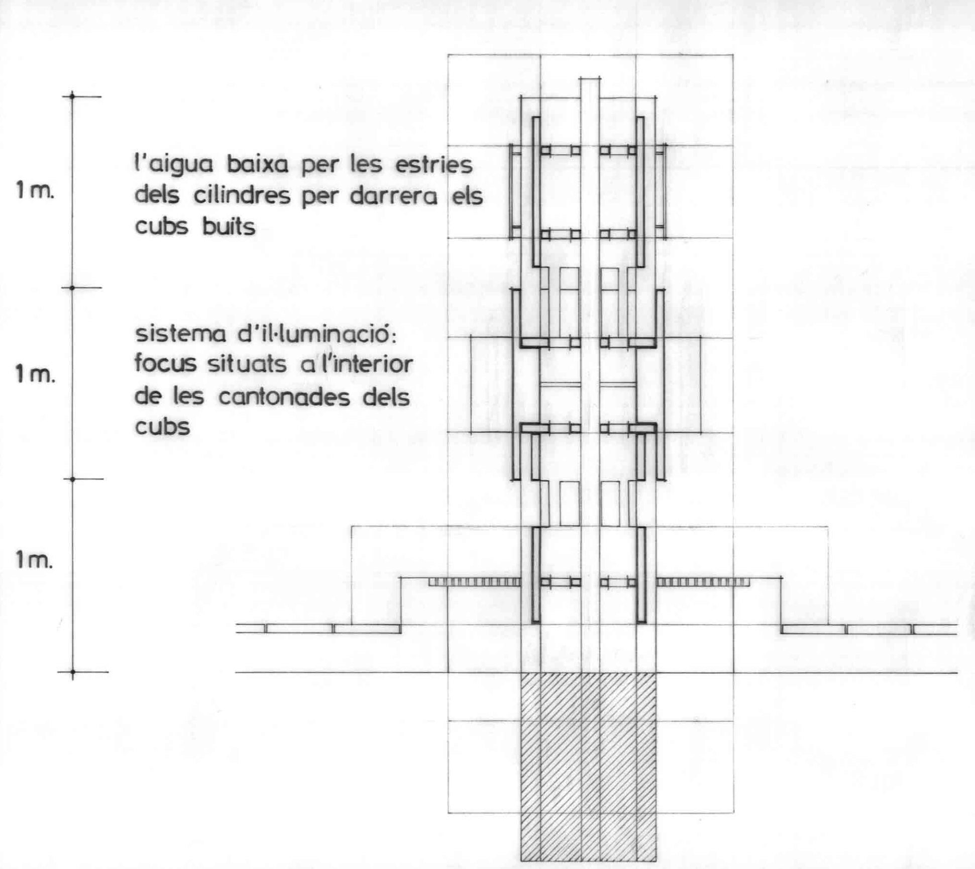
SECCIÓ E: 1/20 sistema funcionament d'aigua en els diferents nivells o pisos del castell
